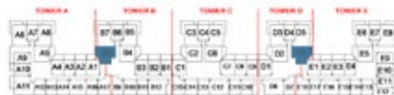
LEVEL 2,4,6
